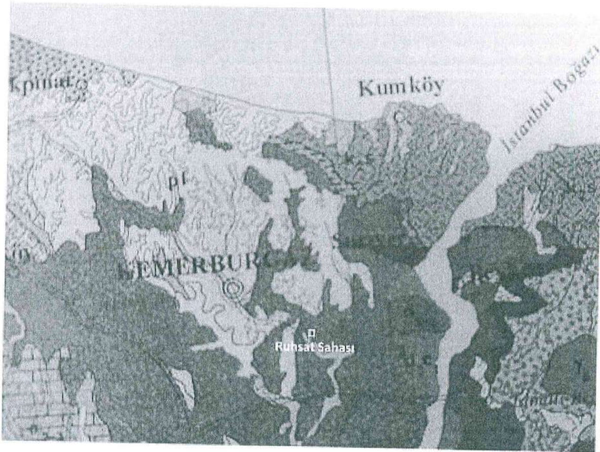
Şekil 8. Ruhsat sahası ve yakın civarını kapsayan alanının jeolojik birimleri (1/500 000'lik MTA Türkiye Jeoloji Haritası). d_{3-2} : alt-Orta Devoniyen karbonatlar ve kırıntılar; d_3 c_1 : Üst Devoniyen karbonat ve kırıntılar; C: Karbonifer karbonat ve kırıntılar; k_2 s : Üst Senoniyen Kırıntılar ve karbonatlar; pl: Pliyosen karasal,
